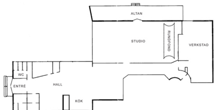
Planritning
